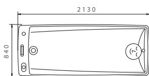
Maße Nassmassagetisch Orient-Alima mit Acryloberteil
