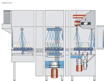
Vista in sezione schematica della macchina
